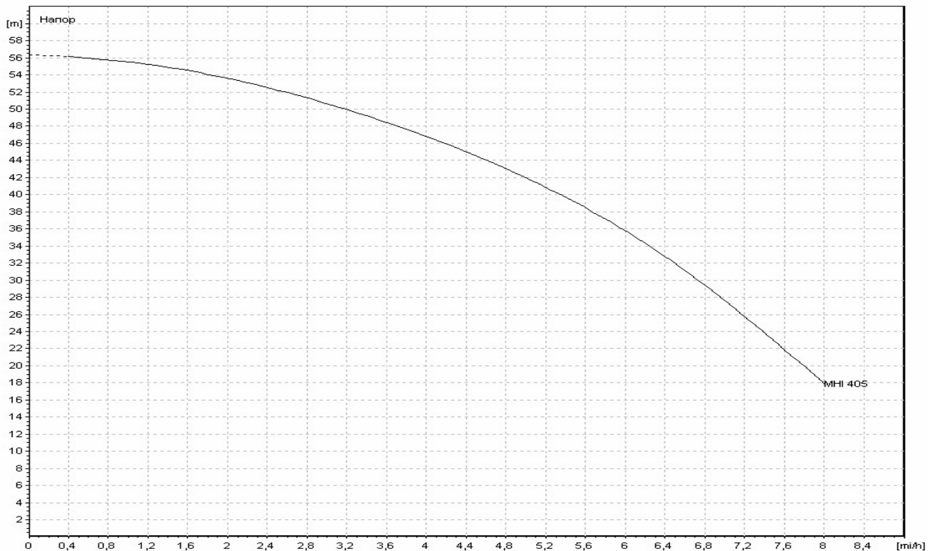
Рабочая линия насоса Wilo MH1 405
